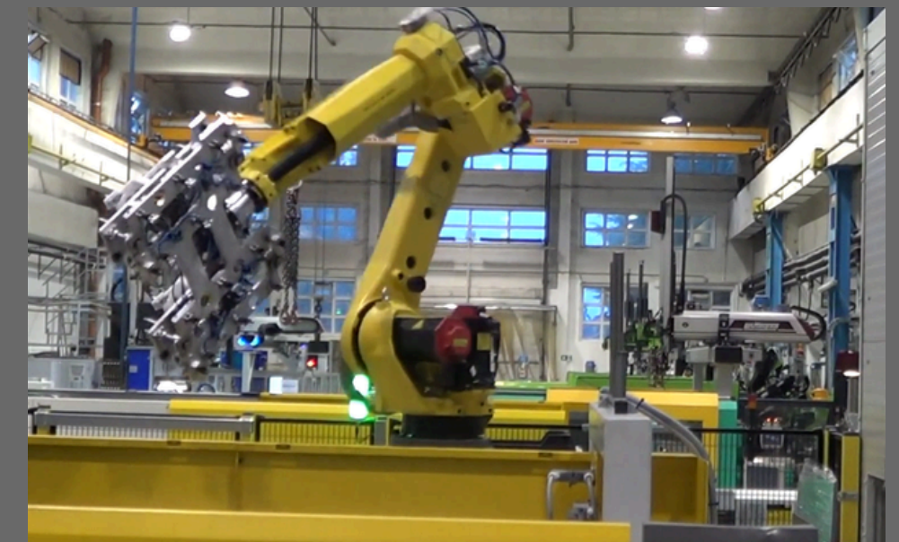
Akkumulátor egység szerelő robotos cella
