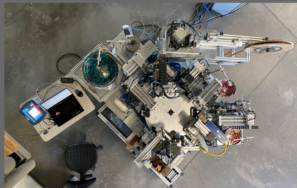
Járműipari csatlakozó körasztalos szerelő
